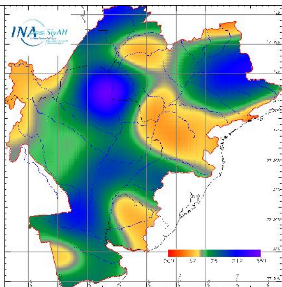
Figura 4a: Anomalías Lluvia Nov/2018
